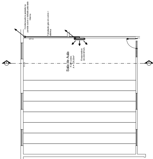
Planta ( Localização da Condensadora e Evaporadora)
