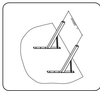
Perspectiva de Fixação do Suporte da Condensadora
