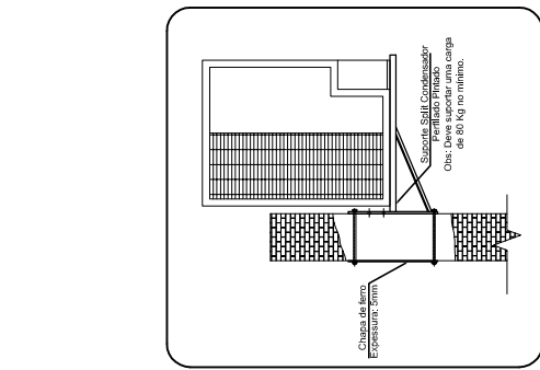
Detalhe da Fixação da Condensadora
