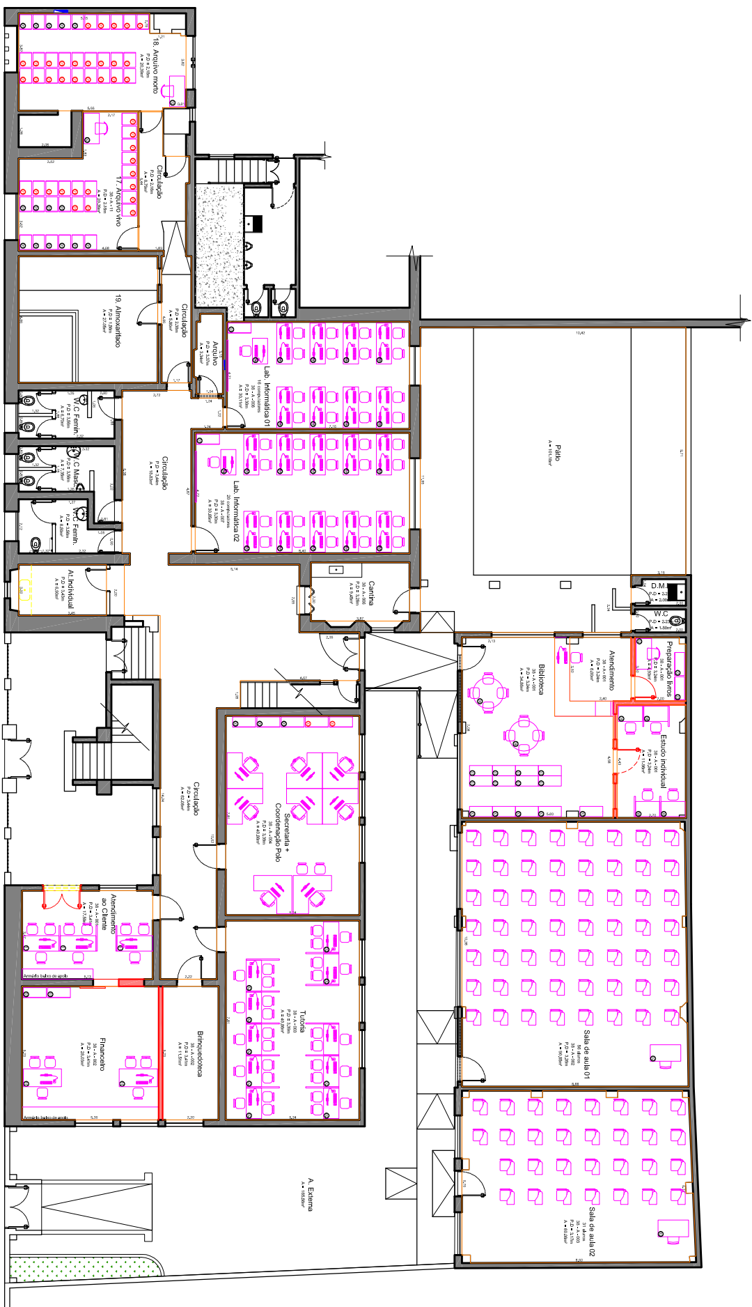
Planta Sub-Solo escala 1:126
